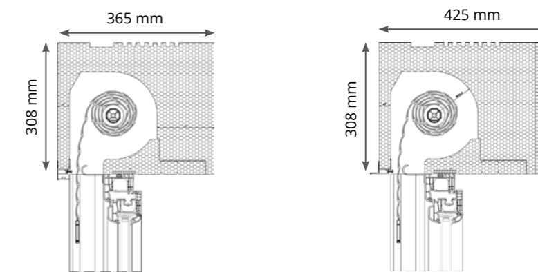
Cassonetto 365 mm.
