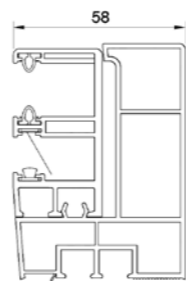
Guida (PVC) singola + MKT* - RS revisione dall'esterno. MK8120 + MK9760
