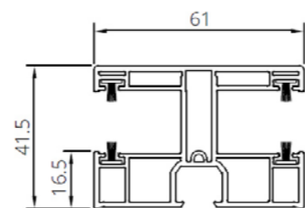
Guida (PVC) singola MAXI. R011309029
