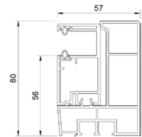
Guida (PVC) singola - RS revisione dall'esterno. MK933 + MK9760
