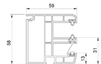
Guida (PVC) singola + MKT* - RS revisione dall'interno. MK8110
