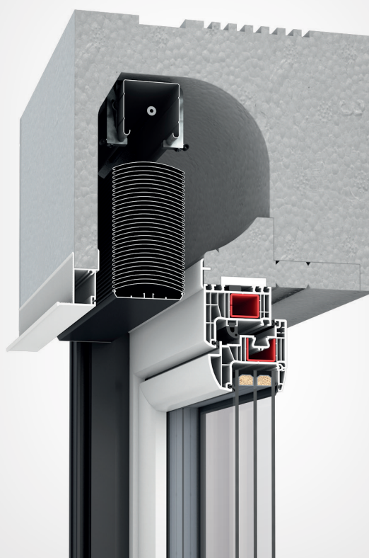
VENEZIANA CON CASSONETTO IN EPS ZS365
