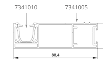
Coulisse unilatérale pour ZF-A, en standard.
