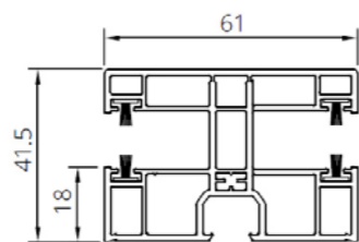
Coulisse (PVC) unilatérale MINI. R0002
