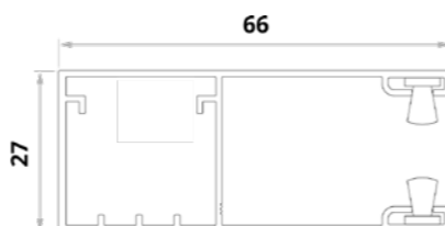
Coulisse unilatérale (pour les lattes H55). PP6600
