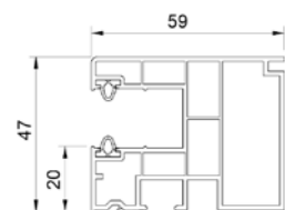
Coulisse (PVC) unilatérale - Trappe de révision RS de l'intérieur.
