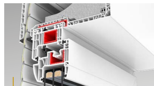
Adaptateur Iglo Energy.
