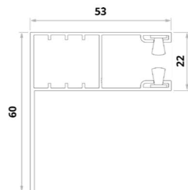
Coulisse angulaire (pour les lattes H37 et H42). 87856
