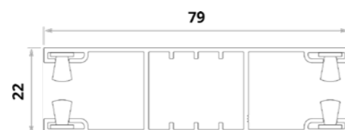
Coulisse bilatérale (pour les lattes H37 et H42). 87858
