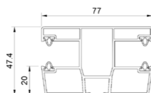
Coulisse (PVC) divisible - Trappe de révision RS de l'intérieur.
