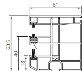
Coulisse (PVC) bilatérale + MKT*. R0003
