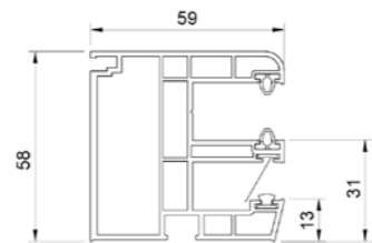
Einseitige Führungsschiene (PVC) + INS* - RS Revision von innen. MK8110
